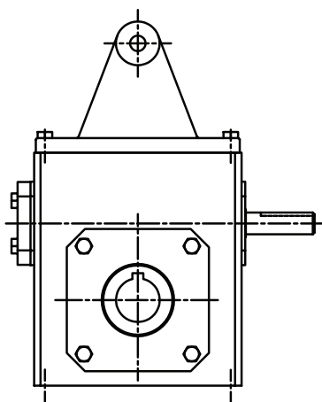
Torque Arm 133 - 325
